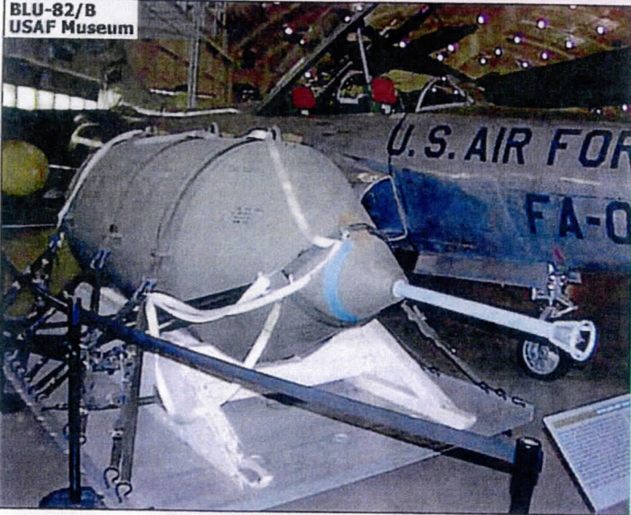
Hier zie je de BLU-82 op een pallet gemonteerd. Ook de kleine container met de 'cargo extraction parachute' is zichtbaar.
