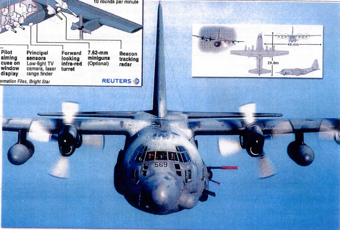
Foto genomen vanuit een KC-135 tankvliegtuig tijdens het bijtanken in de lucht. De verschillende stukken geschut zijn goed te zien aan de rechterkant v.h. toestel.
