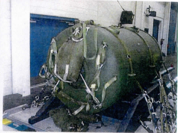
Hier zie je de BLU-82 op een pallet gemonteerd. Ook de kleine container met de 'cargo extraction parachute' is zichtbaar.
